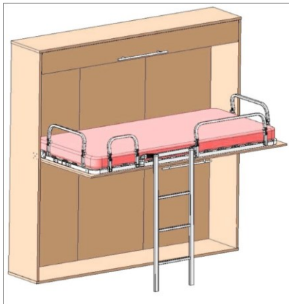
положение «РАЗЛОЖЕНО»
