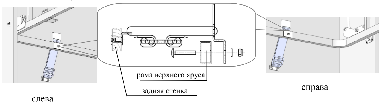
схема установки ремня
